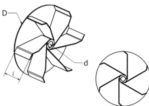
ROTOR - ĽAVÝ: NA OBJEDNÁVKU
