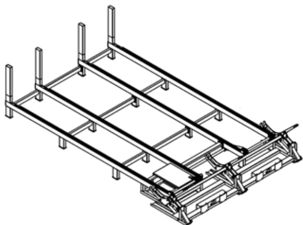
Priečny dopravník guľatiny s nakladačom
