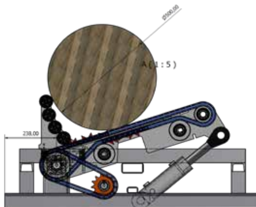
Elektro-hydraulický obracač guľatiny
