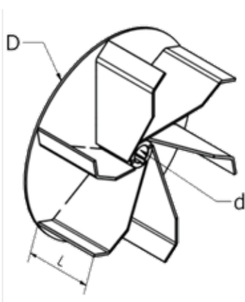
ROTOR - PRAVÝ: ŠTANDARD
