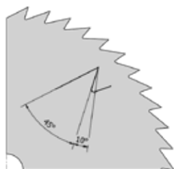
PZ 110 priečne rezanie
