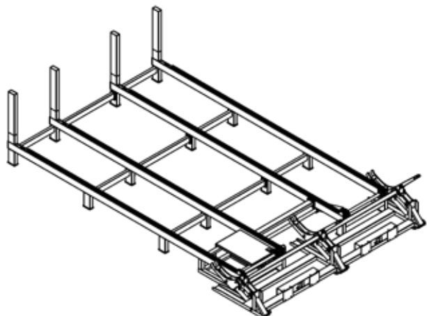
Priečny dopravník guľatiny s nakladačom
