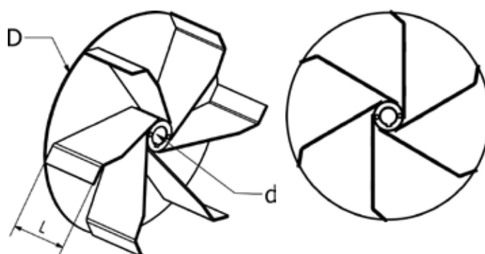
ROTOR - ĽAVÝ: NA OBJEDNÁVKU
