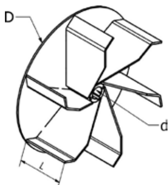
ROTOR - PRAVÝ: ŠTANDARD
